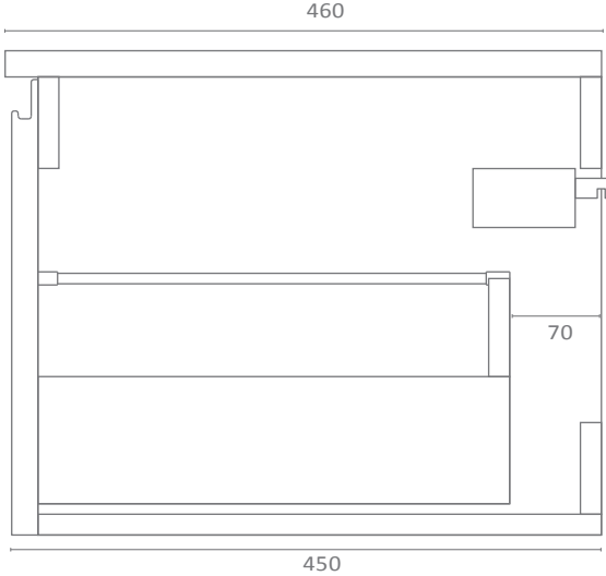
ALZADO DERECHO RIGHT LAY OUT PLAN PROFIL DROIT
