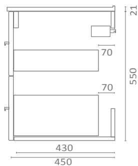
ALZADO IZQUIERDO LEFT LAY OUT PLAN PROFIL GAUCHE
