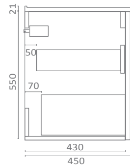
ALZADO DERECHO RIGHT LAY OUT PLAN PROFIL DROIT
