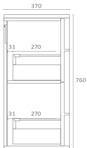
ALZADO MEDIA COLUMNA SEMI COLUMN LAY OUT DEMI COLONNE PLAN PROFIL
