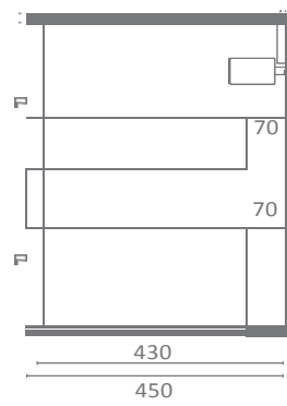
ALZADO IZQUIERDO LEFT LAY OUT PLAN PROFIL GAUCHE
