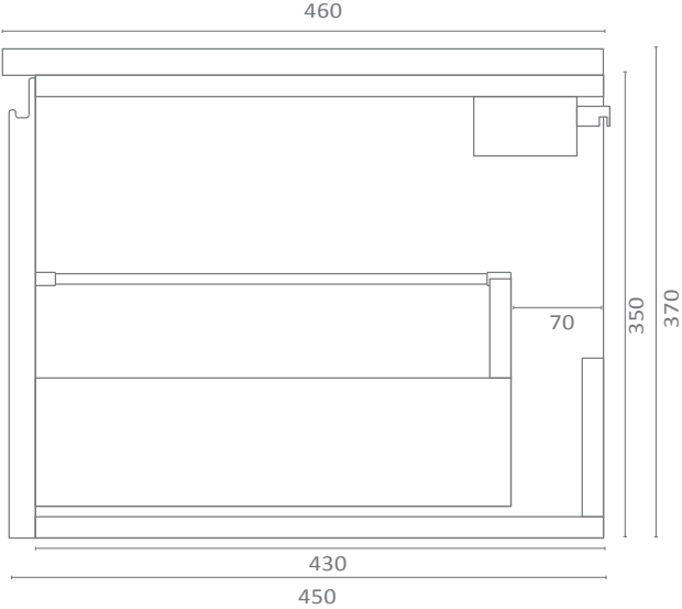
ALZADO DERECHO CUBO CERRADO RIGHT LAY OUT CLOSED CUBO PLAN PROFIL DROIT CUBO FERMÉ
