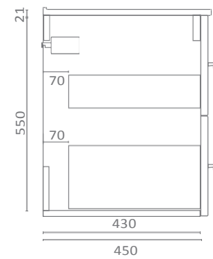
ALZADO DERECHO RIGHT LAY OUT PLAN PROFIL DROIT
