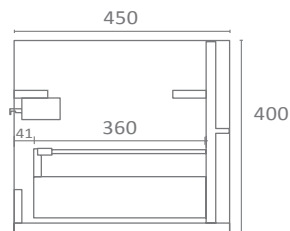
ALZADO LAY OUT PLAN PROFIL
