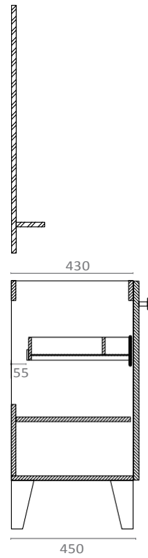
ALZADO DERECHO RIGHT LAY OUT PLAN PROFIL DROIT
