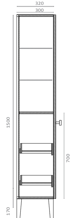
ALZADO DERECHO RIGHT LAY OUT PLAN PROFIL DROIT
